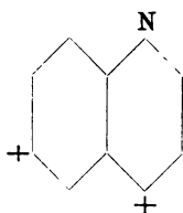
Dahl II.
